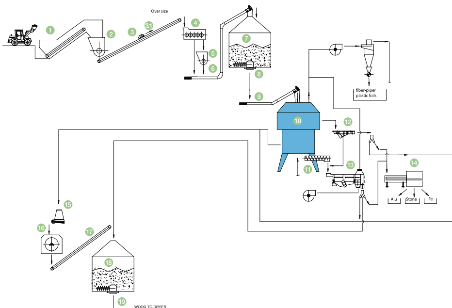
Schema del processo di lavorazione semplificato con l'utilizzo di ORBITAL (in un impianto di produzione di pannello truciolare) Simplified flow-sheet by mean of ORBITAL (in a particle board production line)
