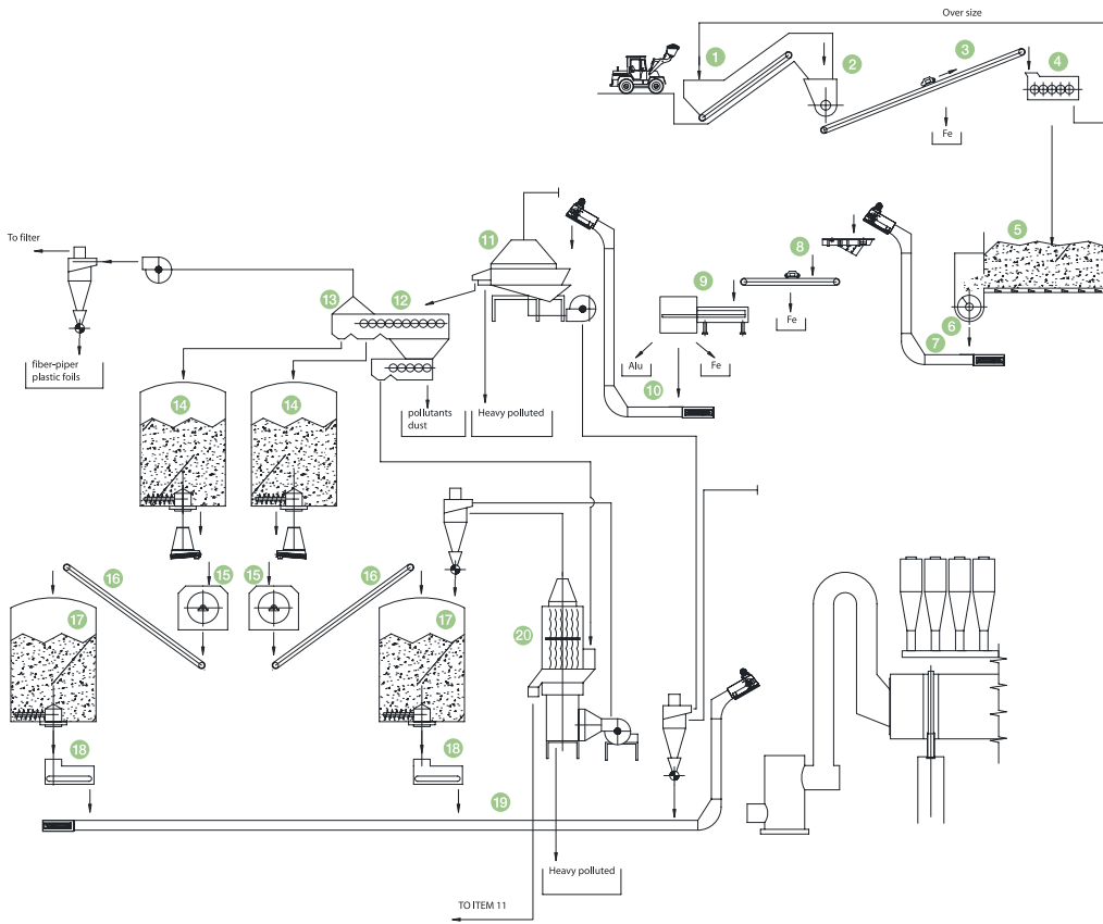
Schema del processo di lavorazione tradizionale (in un impianto di produzione di pannello truciolare) Traditional flow-sheet (in a particle board production line)
